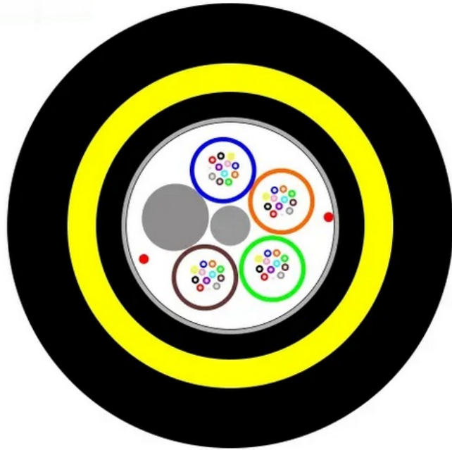
ADSS-D-48F
