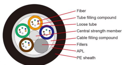
GYTA Fiber Optic Cable
