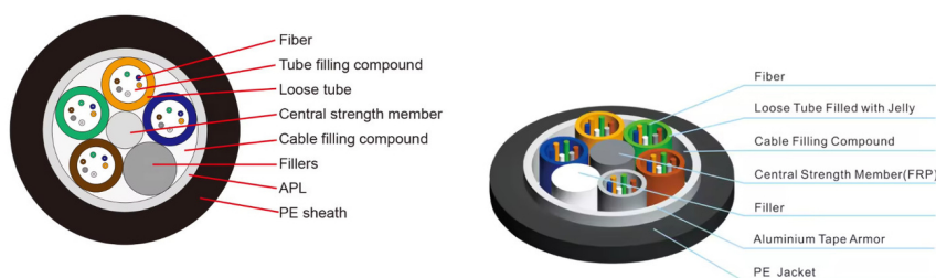
GYTA Fiber Optic Cable
